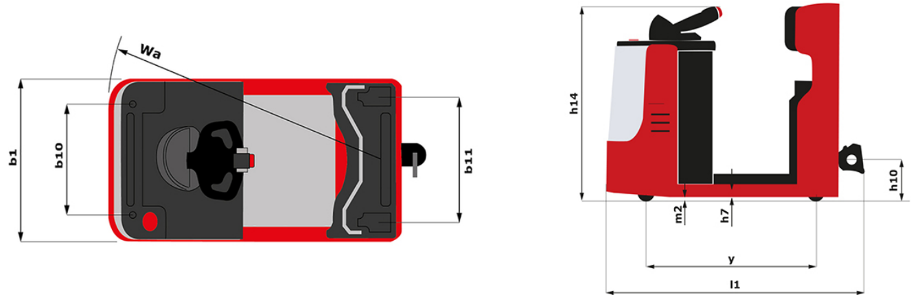
СТ 50 - габаритный чертеж
