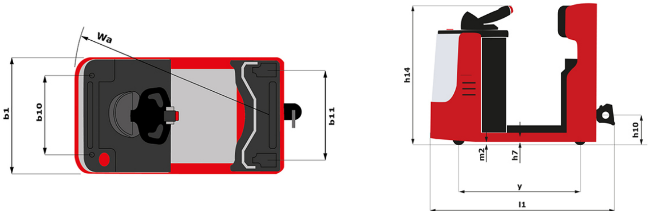
CT 50 - габаритный чертеж
