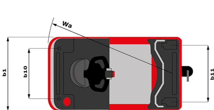
СТ 50 - габаритный чертеж
