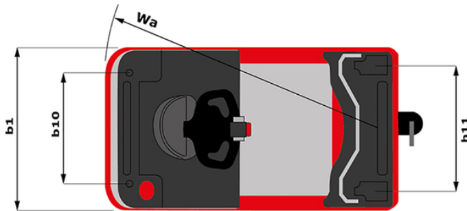
СТ 50 - габаритный чертеж
