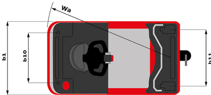
CT 50 - габаритный чертеж
