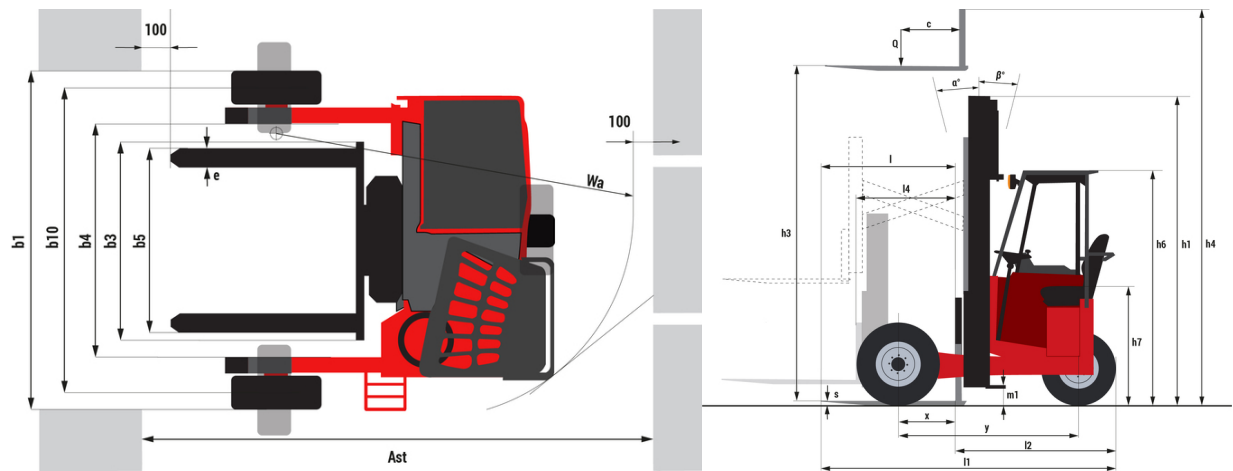
ТММ 20 4W - габаритный чертеж
