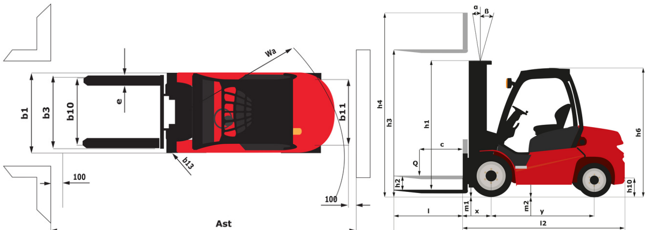
MI-X 70 D - габаритный чертеж
