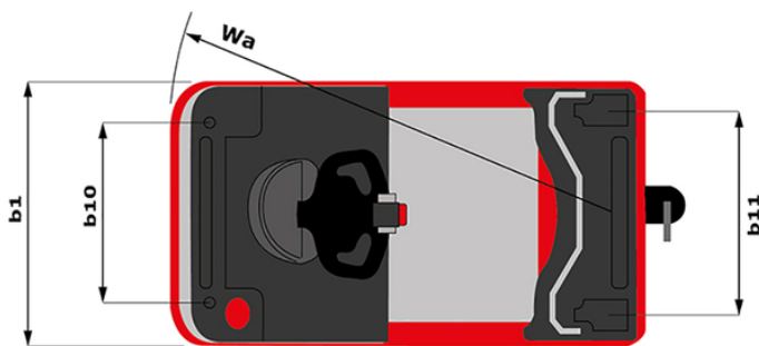
СТ 40 - габаритный чертеж
