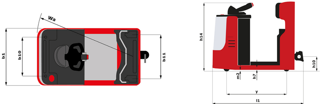
СТ 40 - габаритный чертеж
