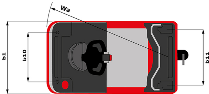
СТ 30 - габаритный чертеж
