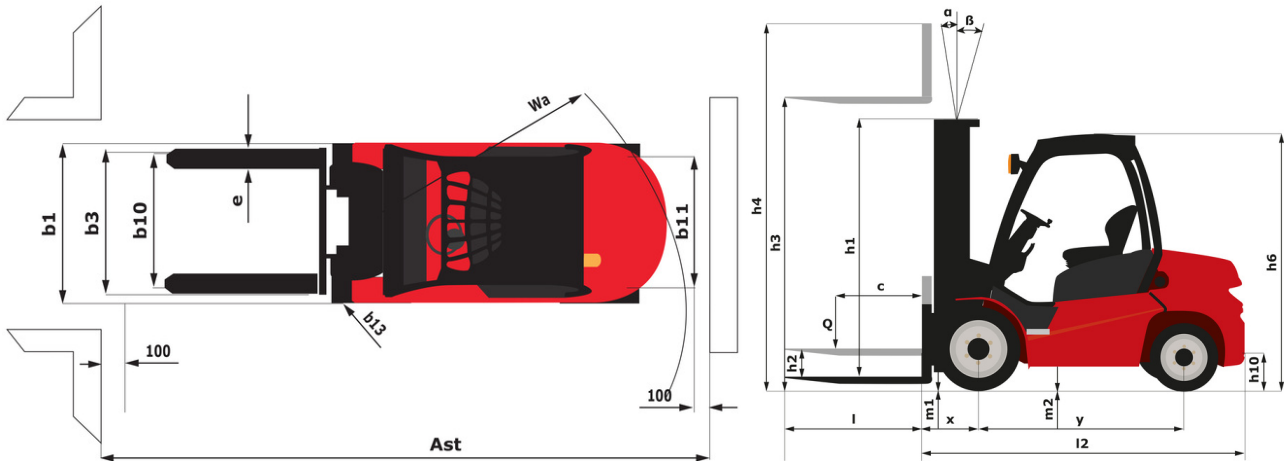
MI 45 G - Rysunek wymiarowy
