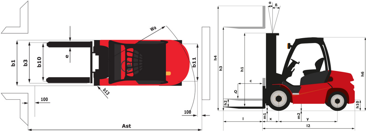
MI 50 D - Diagrama dimensional
