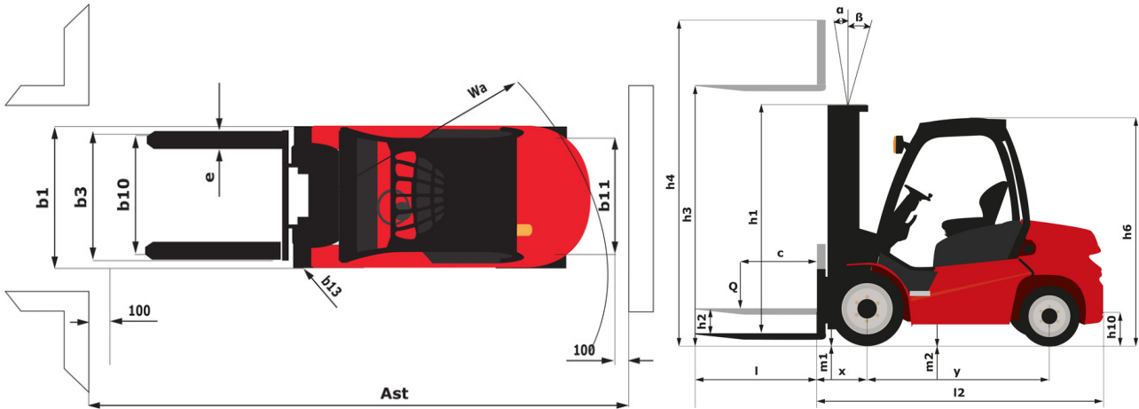
MI 50 D - Tekening met afmetingen
