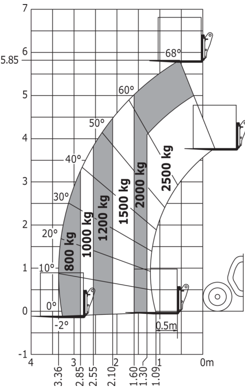
Máquina sobre rodas com garfos
