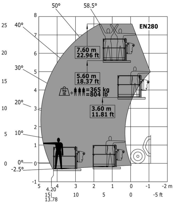
Máquina com cesto para homem - Métrico
