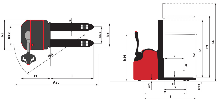
ES 616 LI (5pts) - габаритный чертеж
