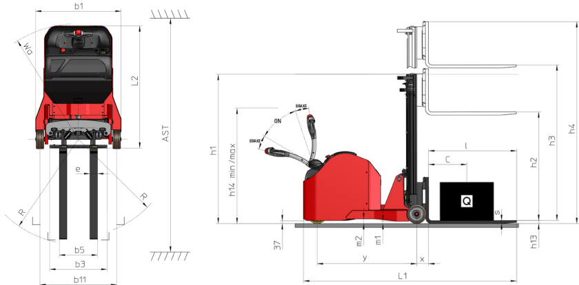
ES-C 711 - Diagrama dimensional
