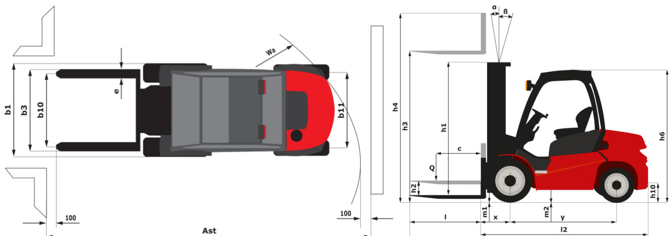
MSI 25 ST5 - Rysunek wymiarowy
