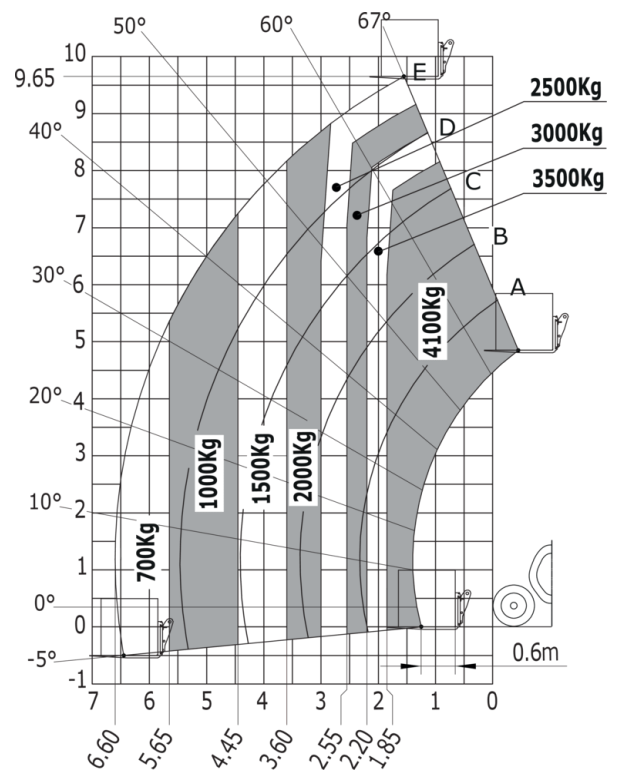
Machine sur pneus avec fourches LC 600 mm Méric
