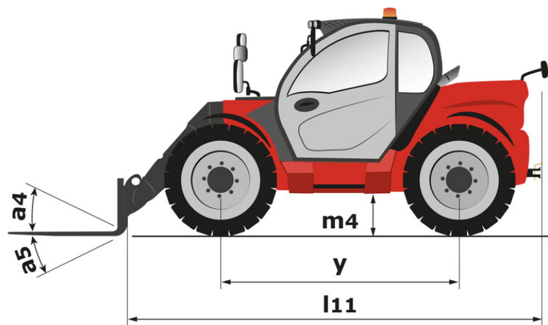
MLT 733-115 - Rysunek wymiarowy
