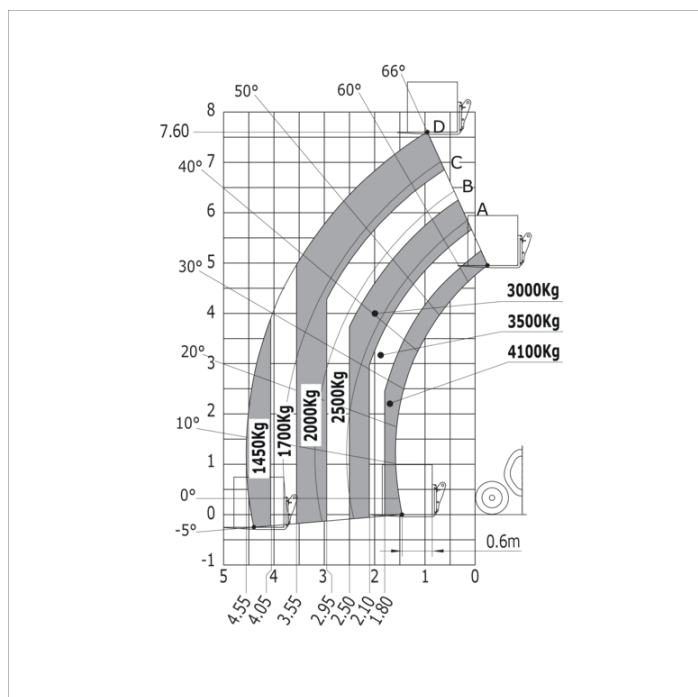
Maszyna na kołach z widłami LC 600 mm
