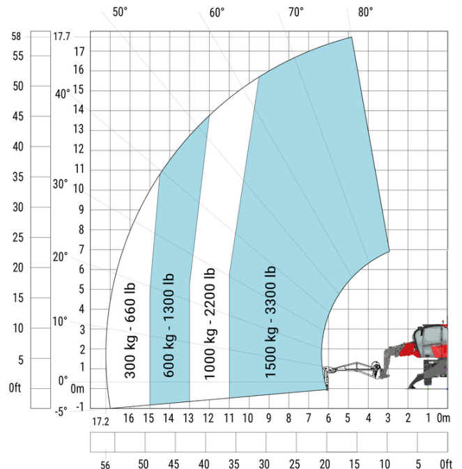
Máquina sobre estabilizadores rebajados con plumín de 1.500 kg con cabestrante (sistema métrico)
