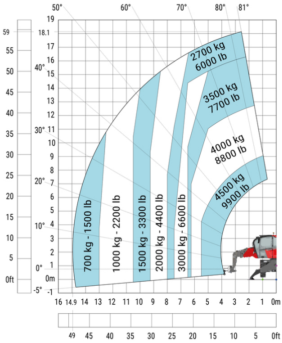
Maszyna na opuszczonych stabilizatorach z hakiem 5000 kg (metryczne)
