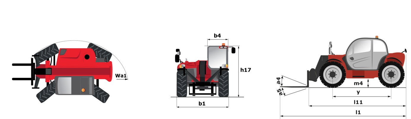
МХТ 1740 Р - габаритный чертеж
