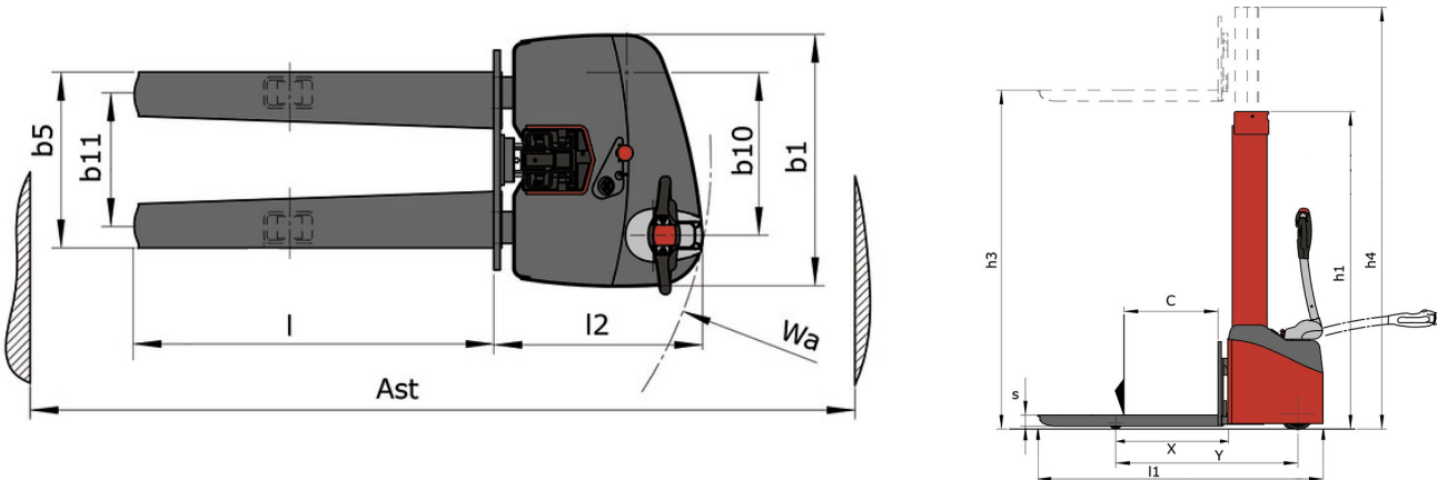
Stacky 10 D28 - Esquemas dimensionais
