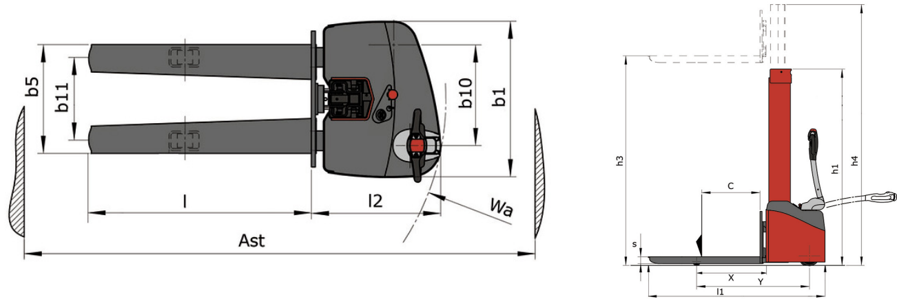
Stacky 10 D28 - Rysunek wymiarowy
