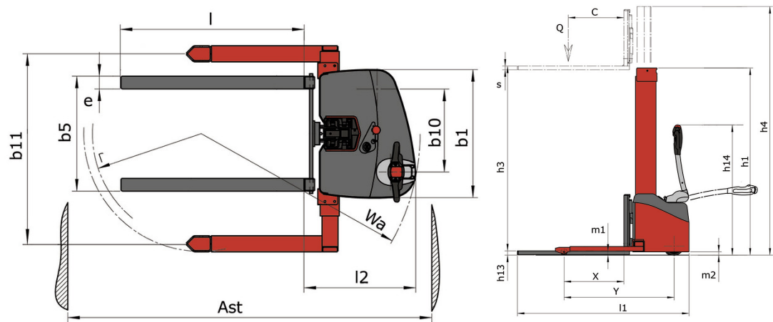
Stacky 10 S16 LE - габаритный чертеж
